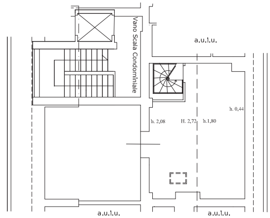
PIANO SOTTOTETTO H=VAR.
